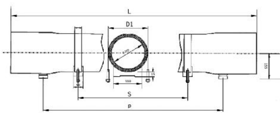
8''侧联反渗透膜壳安装示意图
